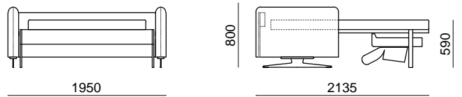
WENDY 30 2,5sed OP
