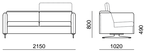
WENDY 30 3sed OP
