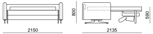
WENDY 30 3sed OP
